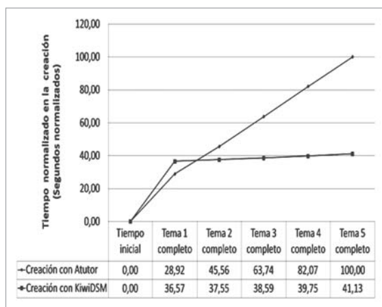
Figura 9. Comparación de tiempos entre la creación de módulos usando la plataforma Atutor Vs la creación de módulos con la herramienta KiwiDSM.
