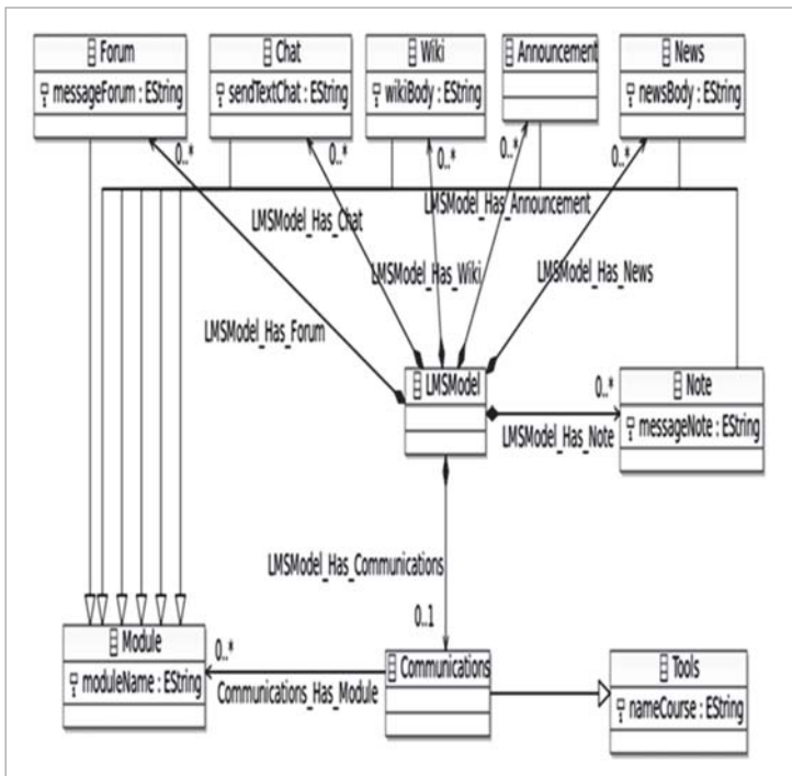
Figura 4. Metamodelo para módulos de comunicaciones de un LMS.
