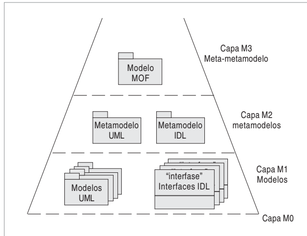
Figura 2. Arquitectura de Metadatos en MOF
