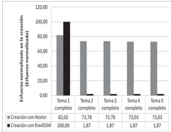
Figura 10. Comparación de usabilidad (esfuerzo) entre la creación de módulos usando la plataforma Atutor y la creación de módulos usando la herramienta KiwiDSM.
