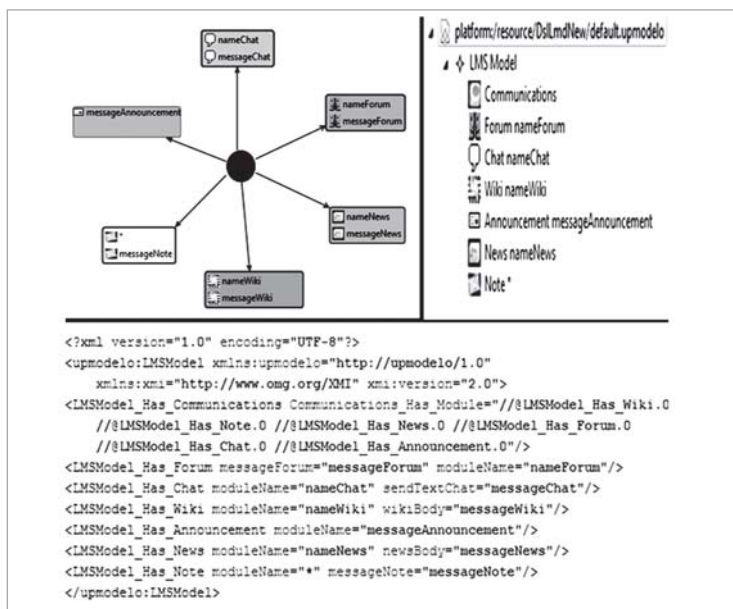
Figura 7. Modelo generado con KiwiDSM y su correspondencia con XMI.
