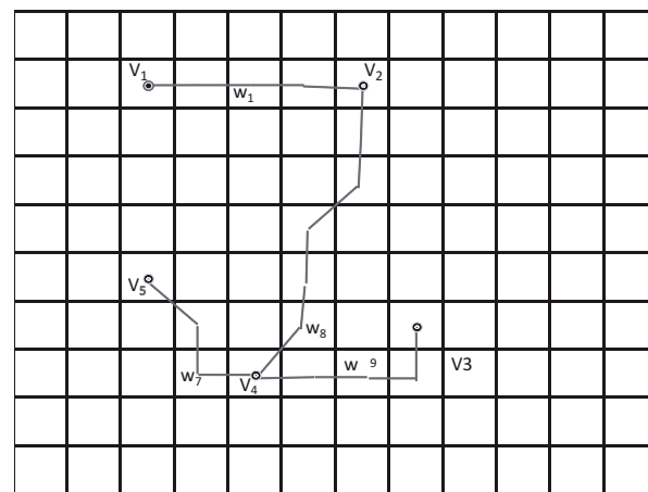
Figura 9. Red vial establecida mediante el algoritmo de Kruskal, árbol de mínima expansión
