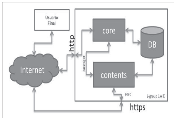
Fig. 6. Topología Framework – ONYX.
